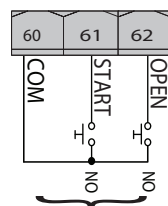
Управление
