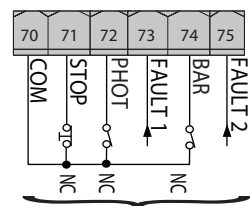
Устройства безопасности
