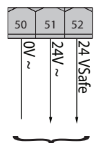
Питание аксессуаров
